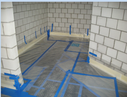
Bodenfläche im Lager mit PE-Folie abgedichtet, Randstellstreifen an den Wänden, bereit zum Einbringen der Bewehrung und zum Betonieren der Lastverteilplatte
