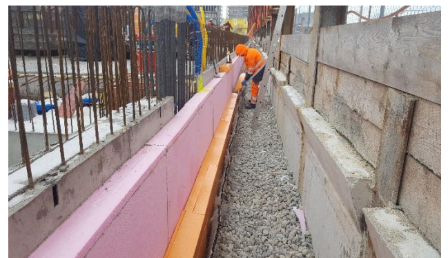
Ende der Montage, wo die letzte Meter Lagerung vor der finalen Hinterfüllung angebracht werden. Links die Wärmedämmung mit der Lagerung (orange) und der Bahnlinie (rechts)
