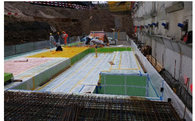
Bei der Ausführung gilt es durch exaktes Arbeiten jede mögliche Körperschallbrücke zu verhindern – nur so bringt die Lagerung ihre volle Dämmleistung. Das Bild oben zeigt das Dämmen der Rohrleitung der Filter – und des Entnahmekrannens.
