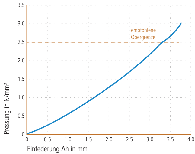
Einfederung
