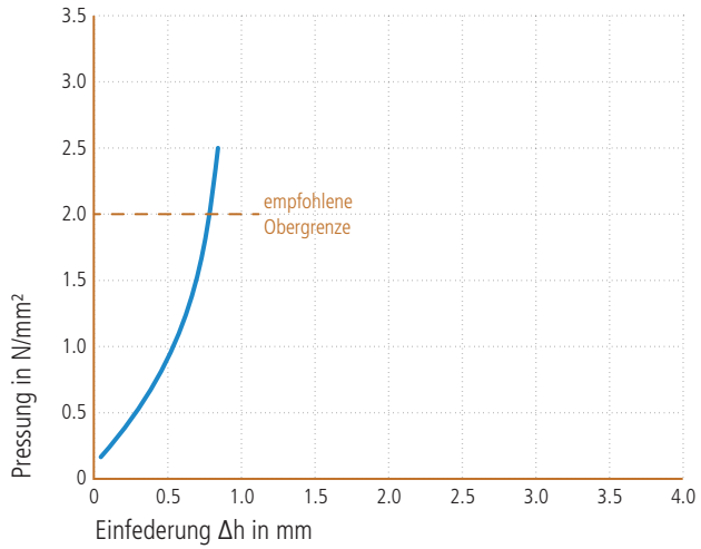
Einfederung
