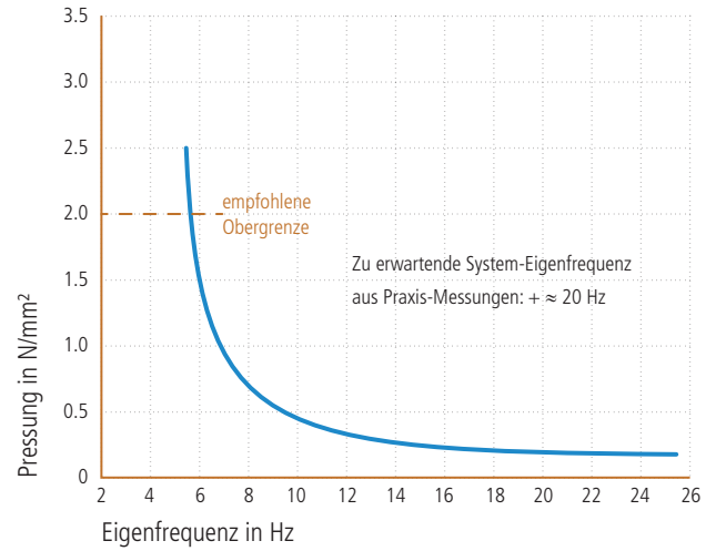
Eigenfrequenz
