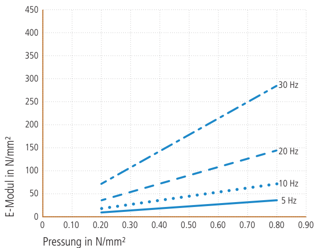
Dynamischer Elastizitätsmodul
