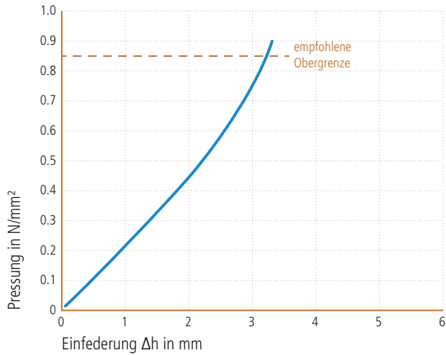
Einfederung
