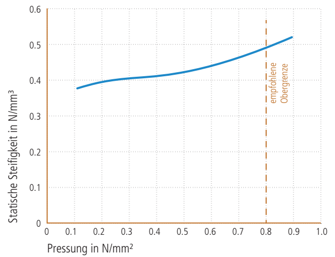
Statische Steifigkeit
