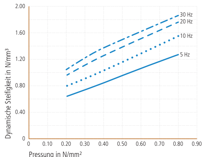
Dynamische Steifigkeit
