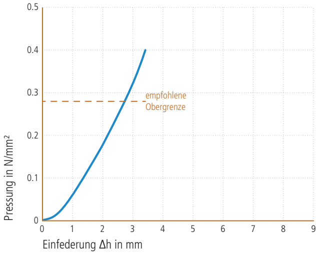
Einfederung
