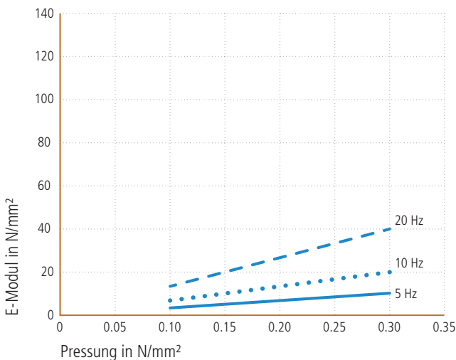
Dynamischer Elastizitätsmodul
