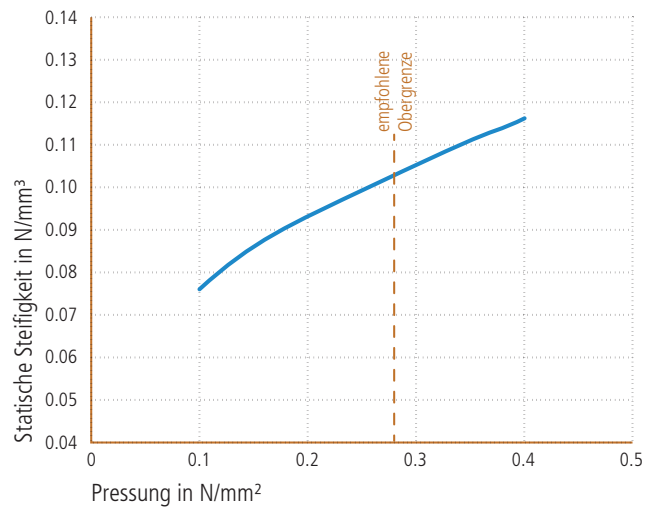
Statische Steifigkeit
