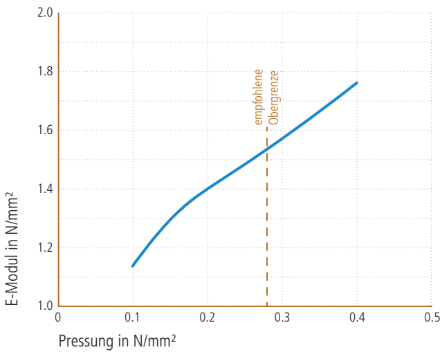
Statischer Elastizitätsmodul
