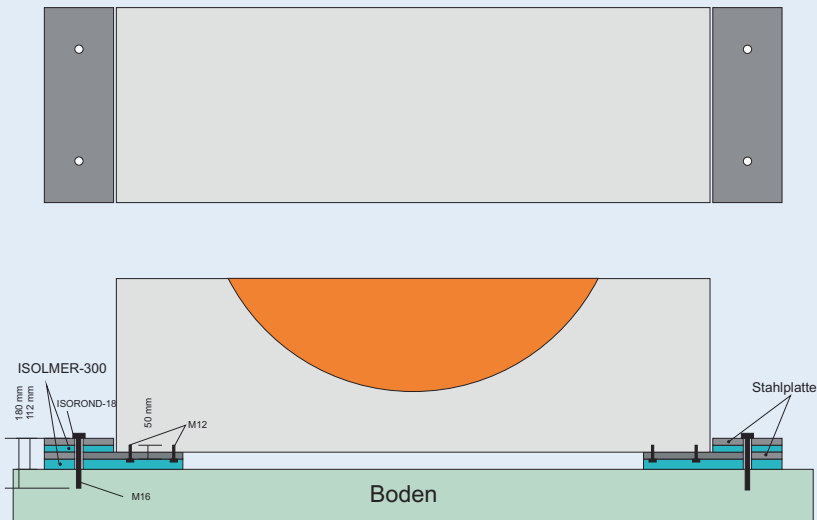
Schematische Darstellung der Lagerung
